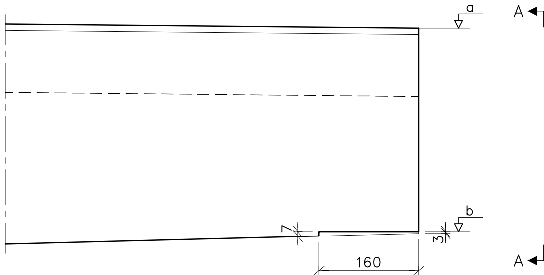
Detalje af TTP ribbeende ved kileudsparring/vederlag
