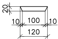
Snit C-C
