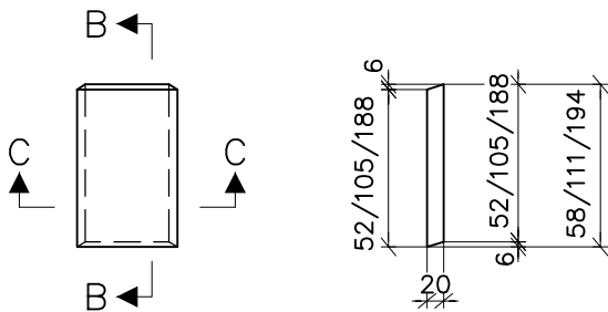
Snit B-B
