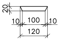
Snit C-C
