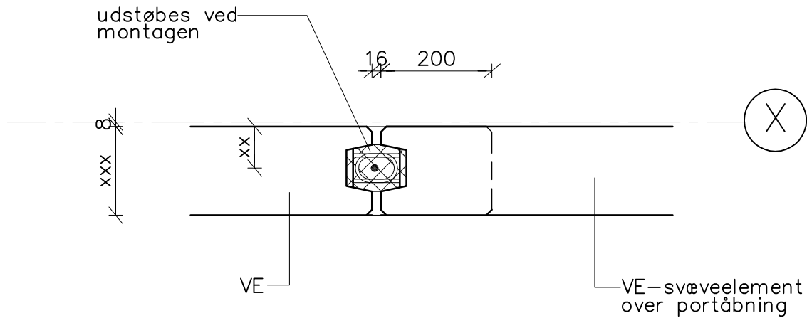
Snit A-A
