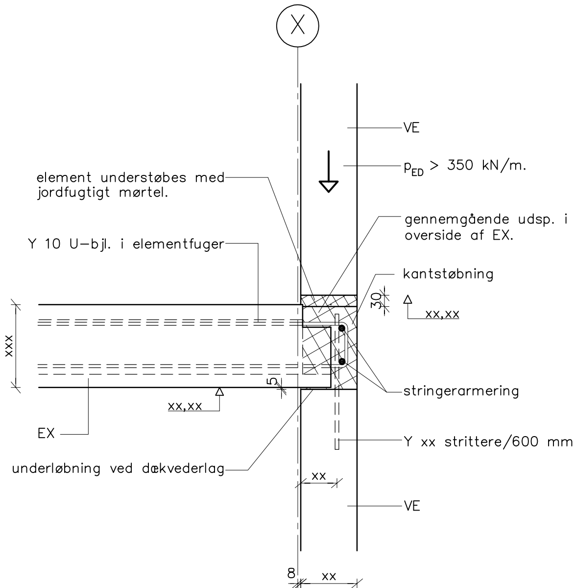
Samling mellem EX / VE (bærende) ved etagekryds.
