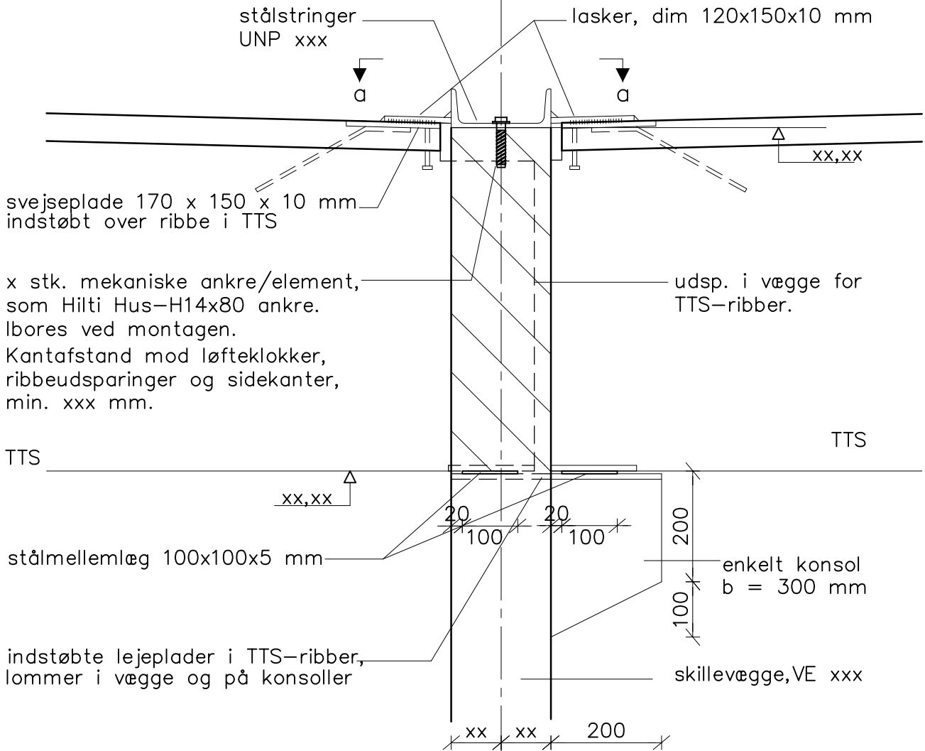
snit a-a
