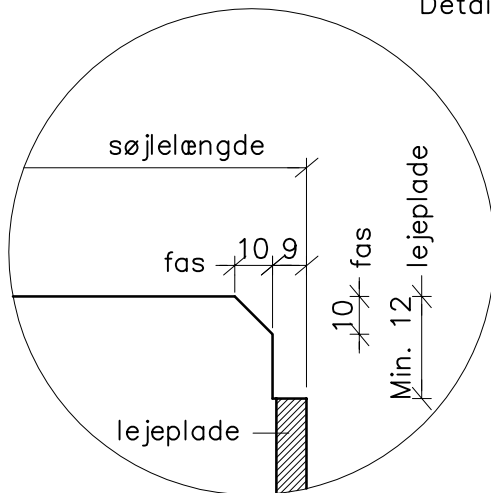
Detail 1 – søjletop, RS
