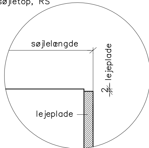
Detail 2 – søjletop, ØS
