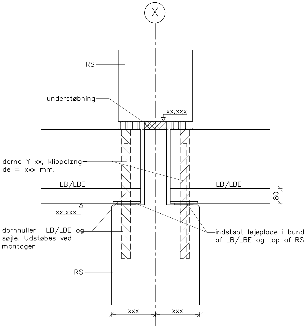
Samling mellem RS/LB og LBE (endesamling – etagekryds)
