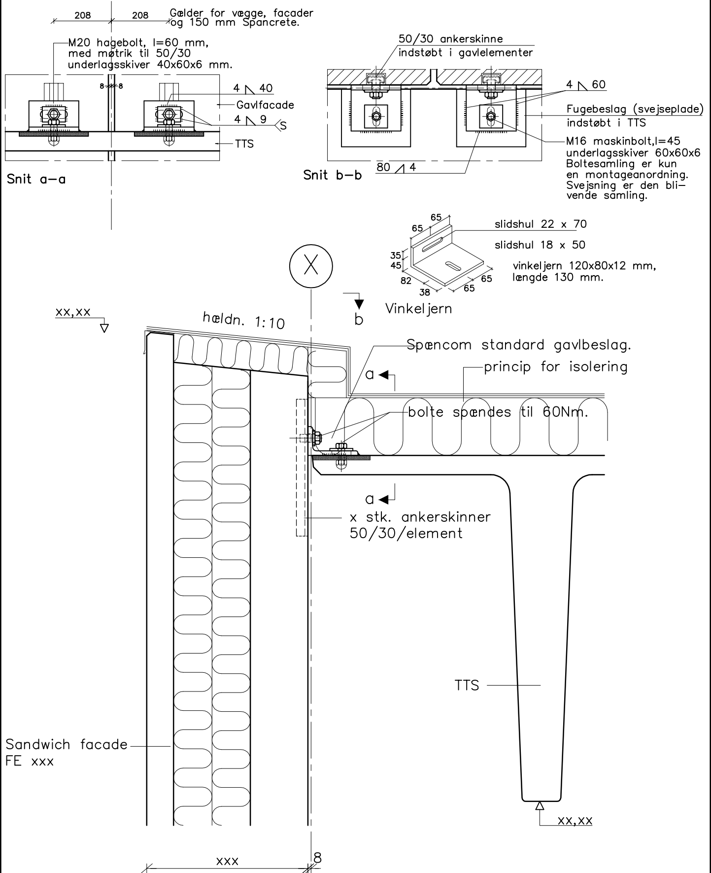
Detailsnit visende samling mellem TTS-tagplader og sandwich facader i gavl.
