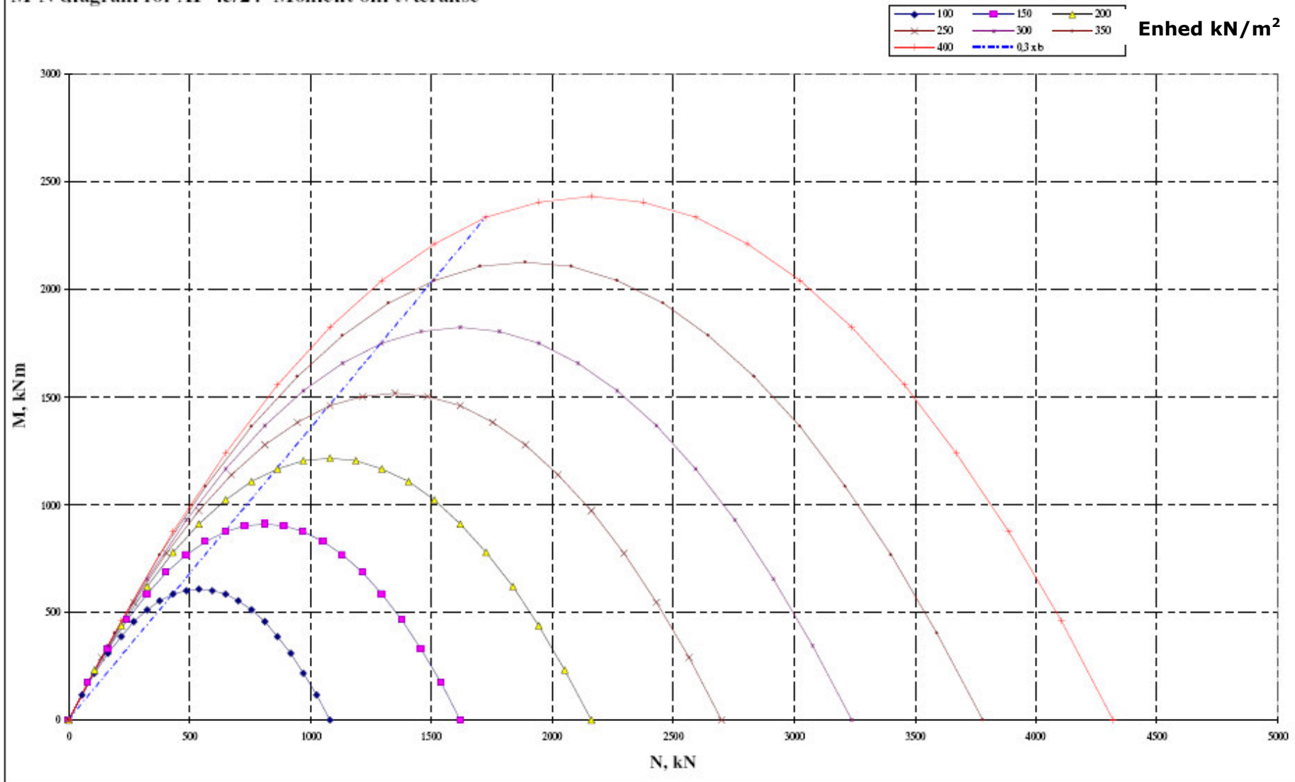
M-N diagram for AF 45/24 Moment om tværsakse
