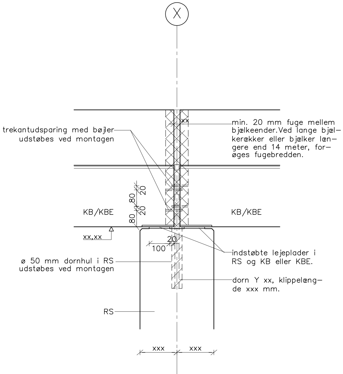
Samling mellem RS / KB/KBE (bøjlesamling)
