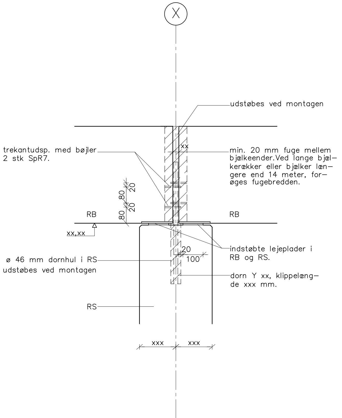
Samling mellem RS / RB-bjælker (bøjlesamling)
