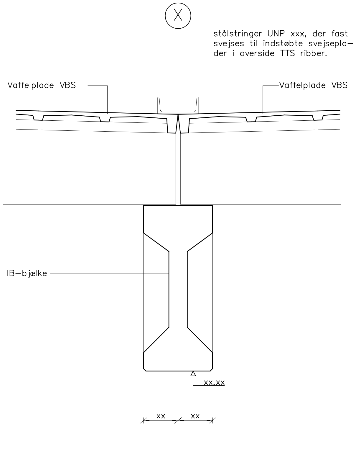
Samling mellem IB/ vaffelplader VBS.
